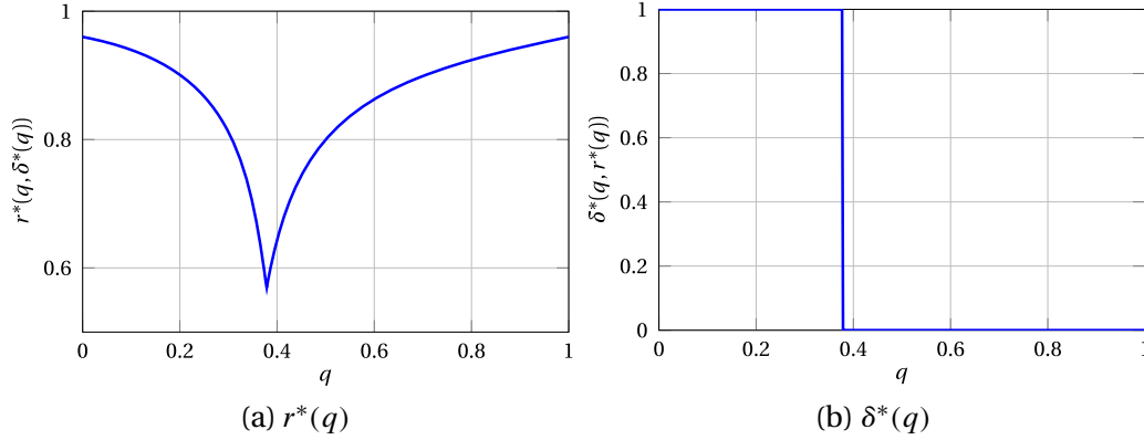
FIGURE S.3. Parameter values: \psi^N = 0.5 , \alpha = 0.5 , \beta = 0.5 , \theta = 0.2 , \sigma = 0.5 , \rho = 0.5 .
